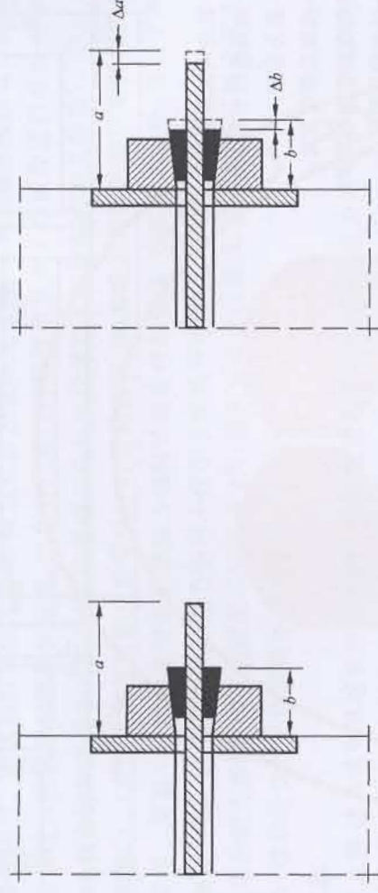
a) 锚固之前,预应力筋顶紧之后
